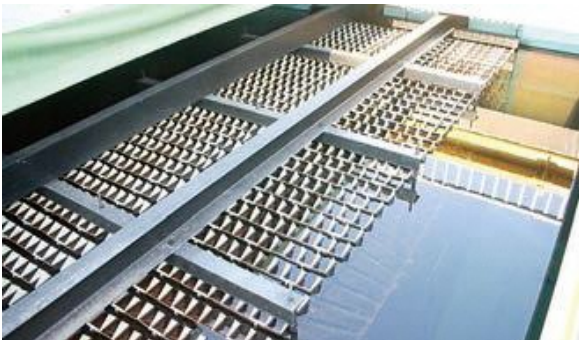
写真 2.4 傾斜板沈澱池
